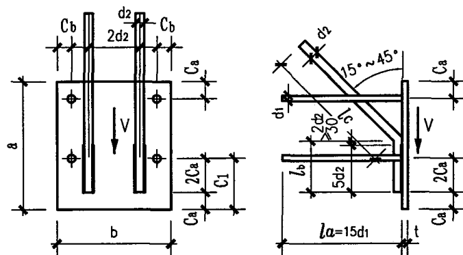
M2-2xx
