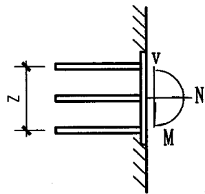
图 G.4.1 拉弯剪作用下的预埋件
