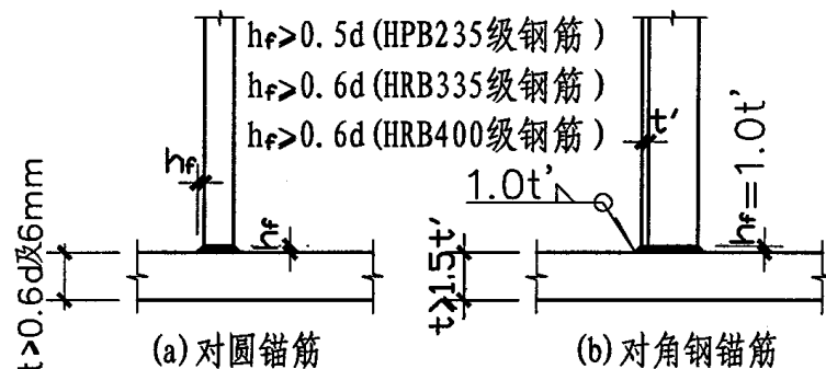
图5.4 T型手工焊的要求
