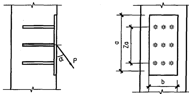
拉剪预埋件
