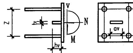
图 G.6.2 带抗剪钢板的压弯剪预埋件
