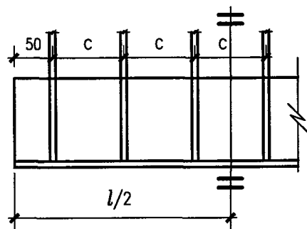
M5-3xx(I) 角钢预埋件
