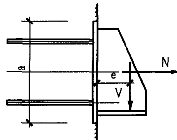
拉弯剪预埋件
