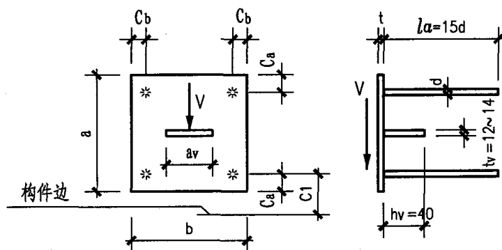
M2-3xx
