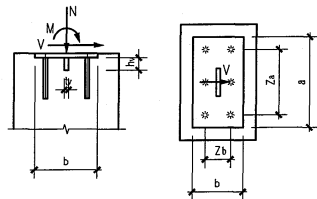
有抗剪钢板的压弯剪预埋件
