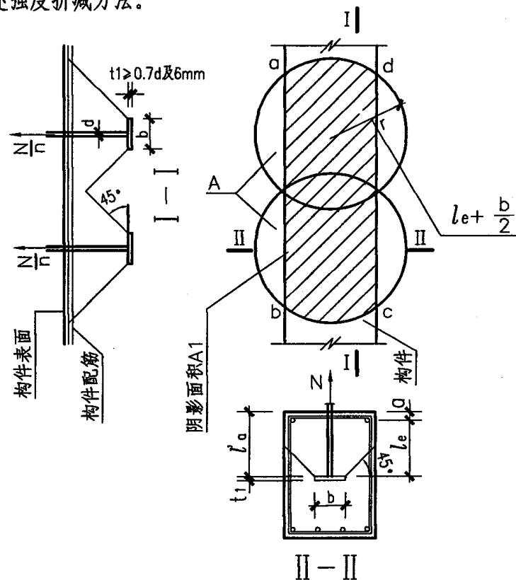
图E.1.3 混凝土截锥体受力图
