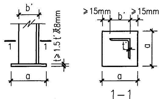
图D.4.2 角钢锚筋端锚板的尺寸
