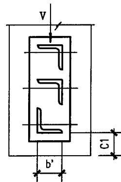
图 G. 3. 4 角钢锚筋的受剪预埋件
