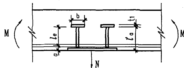
图E.1.2 锚筋端部加焊锚板
