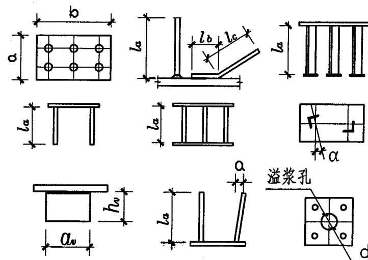
图6.3 预埋件加工
