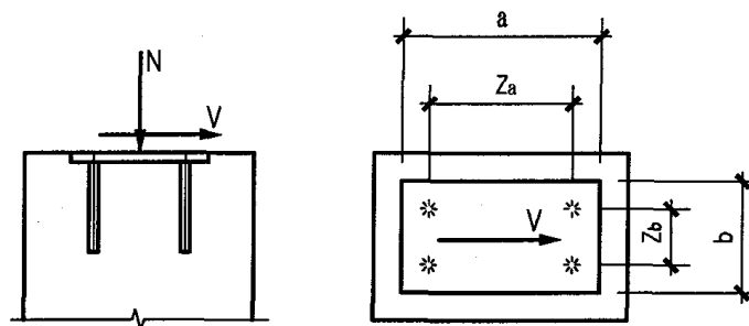
压剪预埋件
