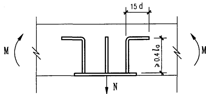
图A.3.3 将锚筋延长到受压区
