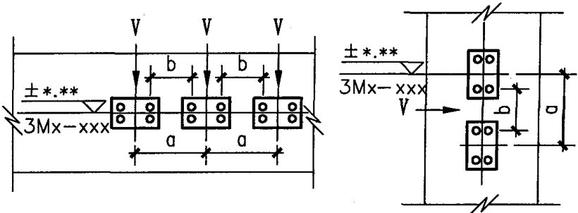
图B.2.2 多块受剪预埋件组合使用
