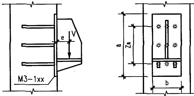
弯剪预埋件(下承式钢牛腿)
