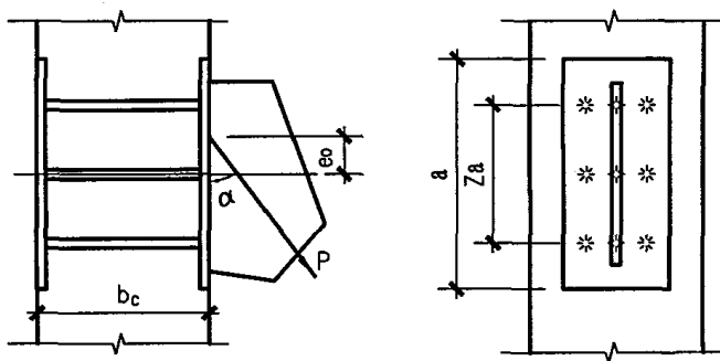
柱间支撑锚筋预埋件
