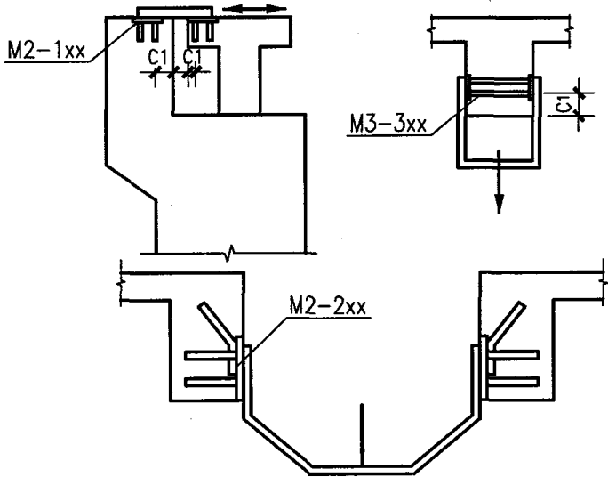
受剪预埋件应用部位举例
