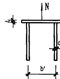
图 G.2.1 直锚筋轴心受拉预埋件
