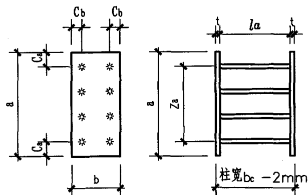
M3-3xx(bc)
