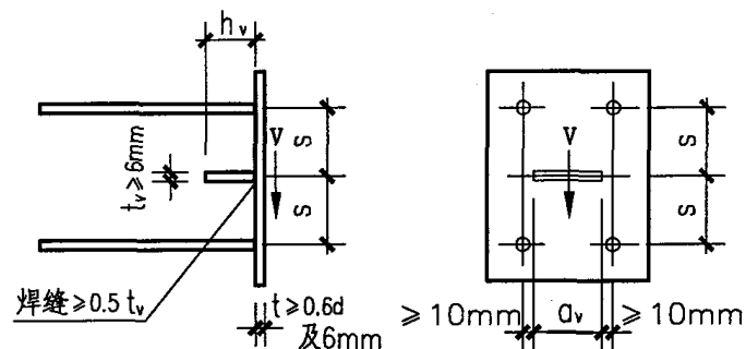
图D.3.4 带抗剪钢板的预埋件
