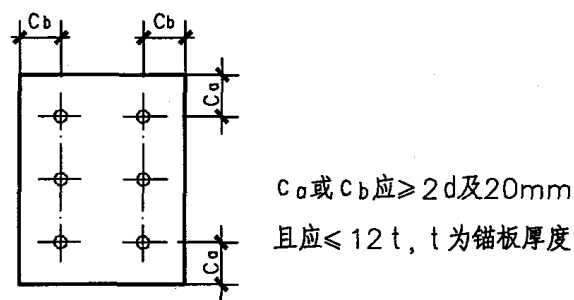
图D.3.1 锚筋到锚板的边距
