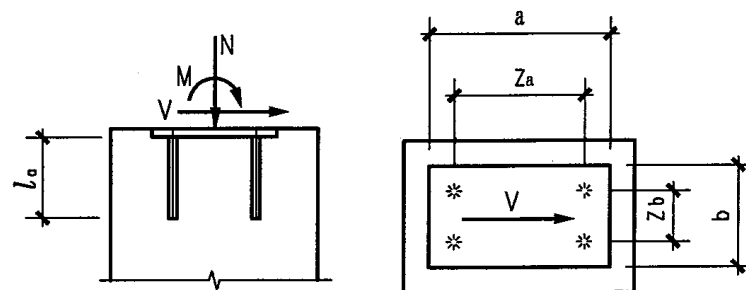
无抗剪钢板的压弯剪预埋件
