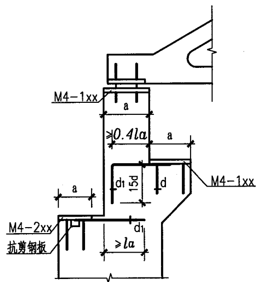
压弯剪预埋件应用部位举例
