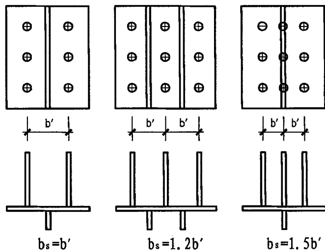
图 G.2.2 锚板弯曲变形的折算宽度
