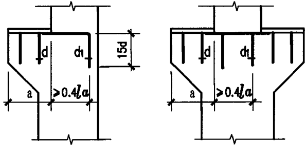
拉筋现场弯折示意图
