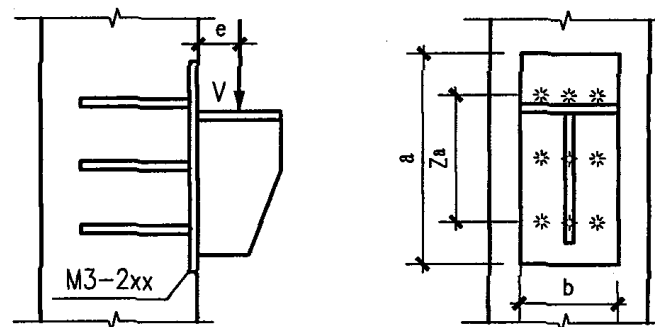
弯剪预埋件(上承式钢牛腿)
