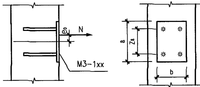
拉弯预埋件
