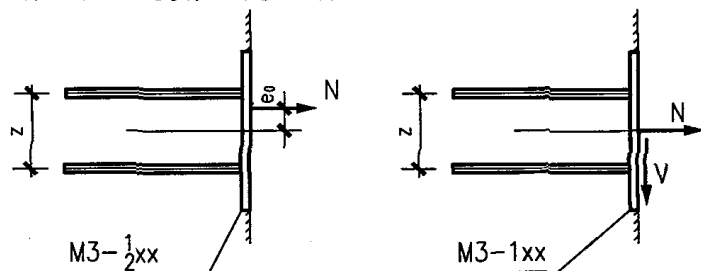
拉弯预埋件
