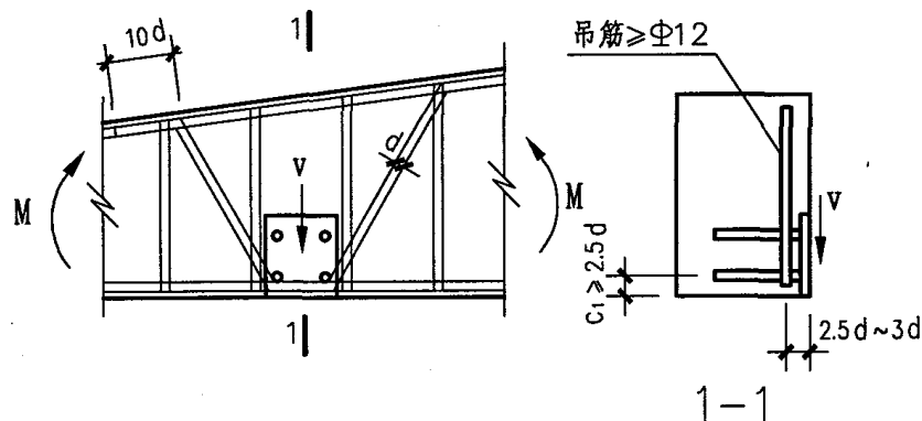
图A.3.4 加吊筋将剪力传至受压区
