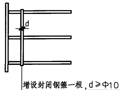
图A.3.5 地震区受力锚筋构造要求
