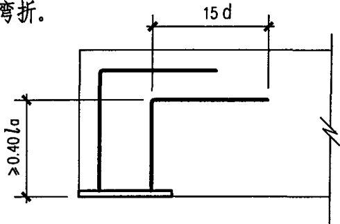
图B.2.3 预埋件受拉锚筋的弯折规定
