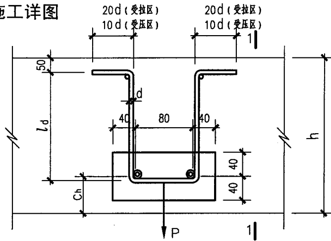
M6-1xx ( box h, Ch)
